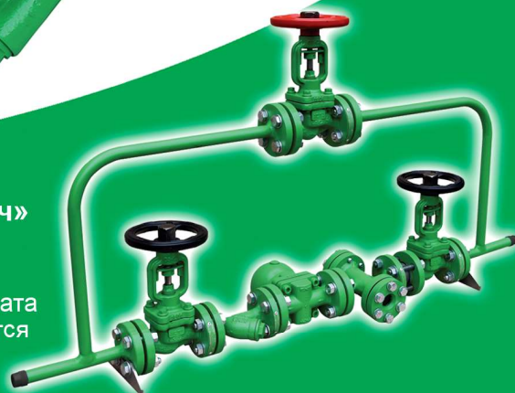
Конденсатоотводчик термодинамический АСТА ТД DN15-50, PN40 фланец/резьба
